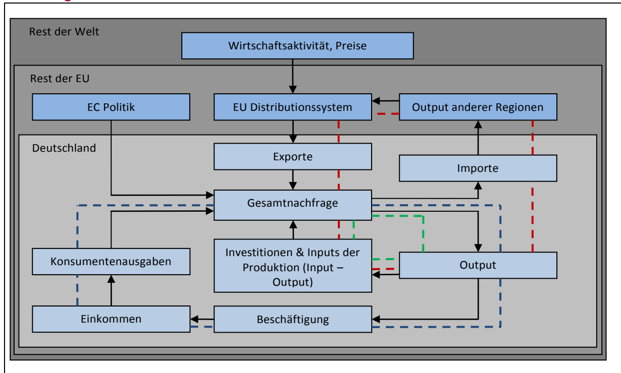
Abbildung 2 E3ME und G3M – Ein ökonomisches Modell für Wirtschaft und Arbeitsmarkt
