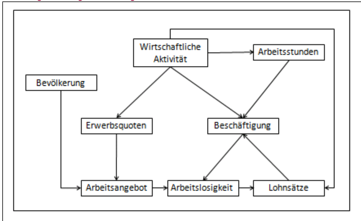
Abbildung 7 Endogene Beziehungen im G3M Modell
